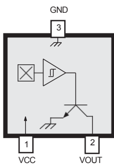
SOT-23-3L
