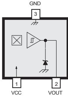
SOT-23-3L (тип M)
