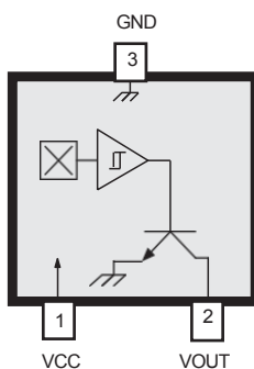
SOT-23-3L (тип М)
