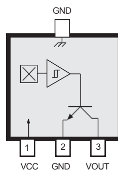
SOT-89 (тип S)
